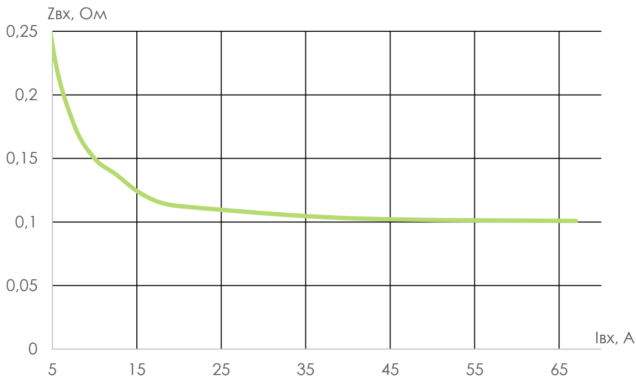
Рисунок 2.3 Полное сопротивление токового входа блока при питании устройства БЗП-01
